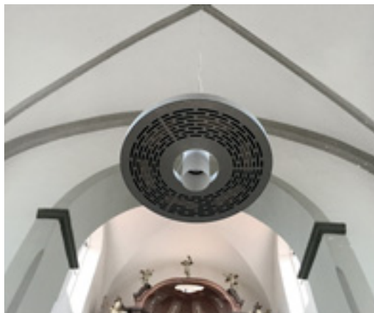
4 Auf dem Weg zum Radstrahler: Der erste Versuch im Dezember 2016, das für die Decken von Produktionshallen entwickelte Heizelement mit einem Leuchtmittel zu kombinieren.
